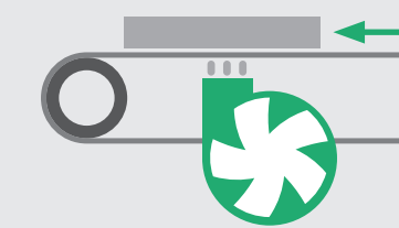
Depressore interno (taratura variabile, inverter) Internal vacuum fan (setting variable, inverter) Imupöytä, puhallin integroitu koneen jalustaan (säädettävissä portaattomasti, invertteri)
