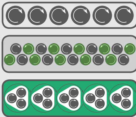
Gruppo spazzole tangenziali / sistema planetario Tangential brushes unit / planetary system Pyörivä harjaysikkö / karuselli-järjestelmä
