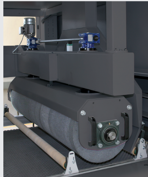
Gruppo spazzola longitudinale Longitudinal brush unit Pitkittäisharjaysikkö
