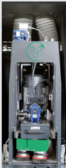
Gruppo spazzole tangenziali / sistema planetario Tangential brushes unit / planetary system Pyörivä harjaysikkö / karuselli-järjestelmä
