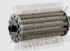
Gruppo spazzola longitudinale Longitudinal brush unit Harjaysykkö
