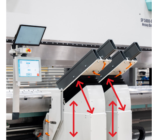
Liike syntyy CNC-ohjatuilla sähkösylintereillä, manuaalinen asetus ei tarpeen
