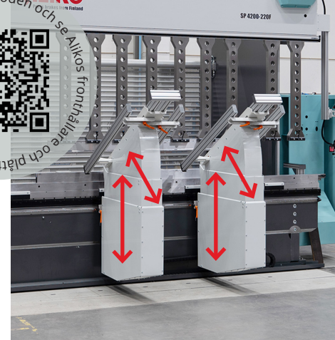
Rörelse med elektriska cylindrar, manuell justering mellan program behövs inte.
