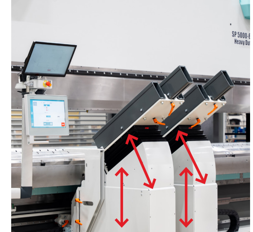
Rörelse med elektriska cylindrar, manuell justering mellan program behövs inte.
