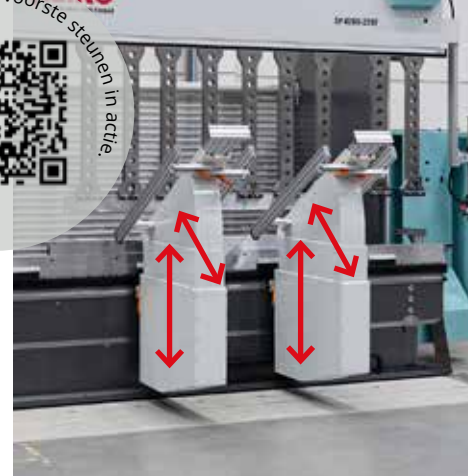
Beweging via CNC-gestuurde elektrische cilinders, geen handmatige instelling nodig
